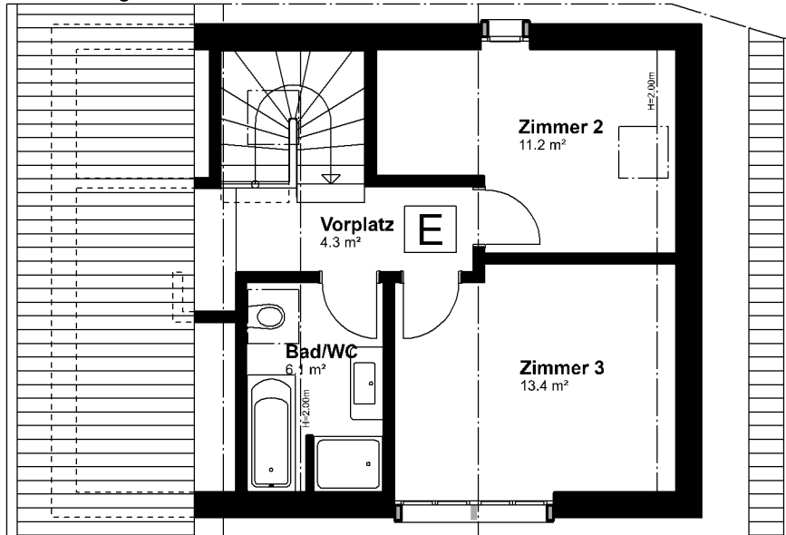
Dachgeschoss
